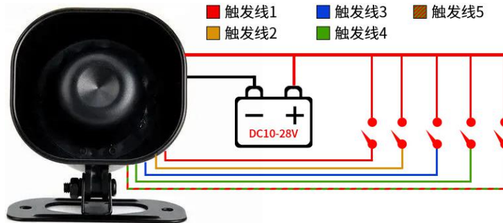
2: 高电平触发单曲播放——接线方式
