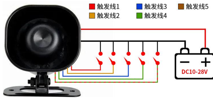
2: 高电平触发单曲播放——接线方式
