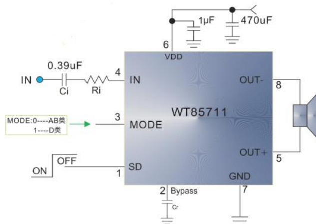
WT85711应用电路图
