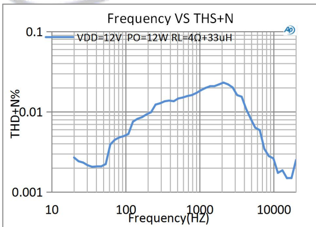
图 3: Frequency VS.TH D+N
